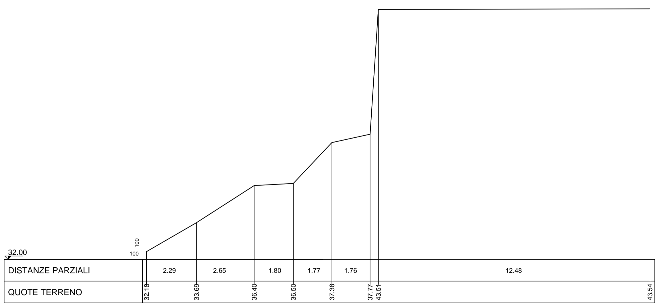
SEZIONE C - C
