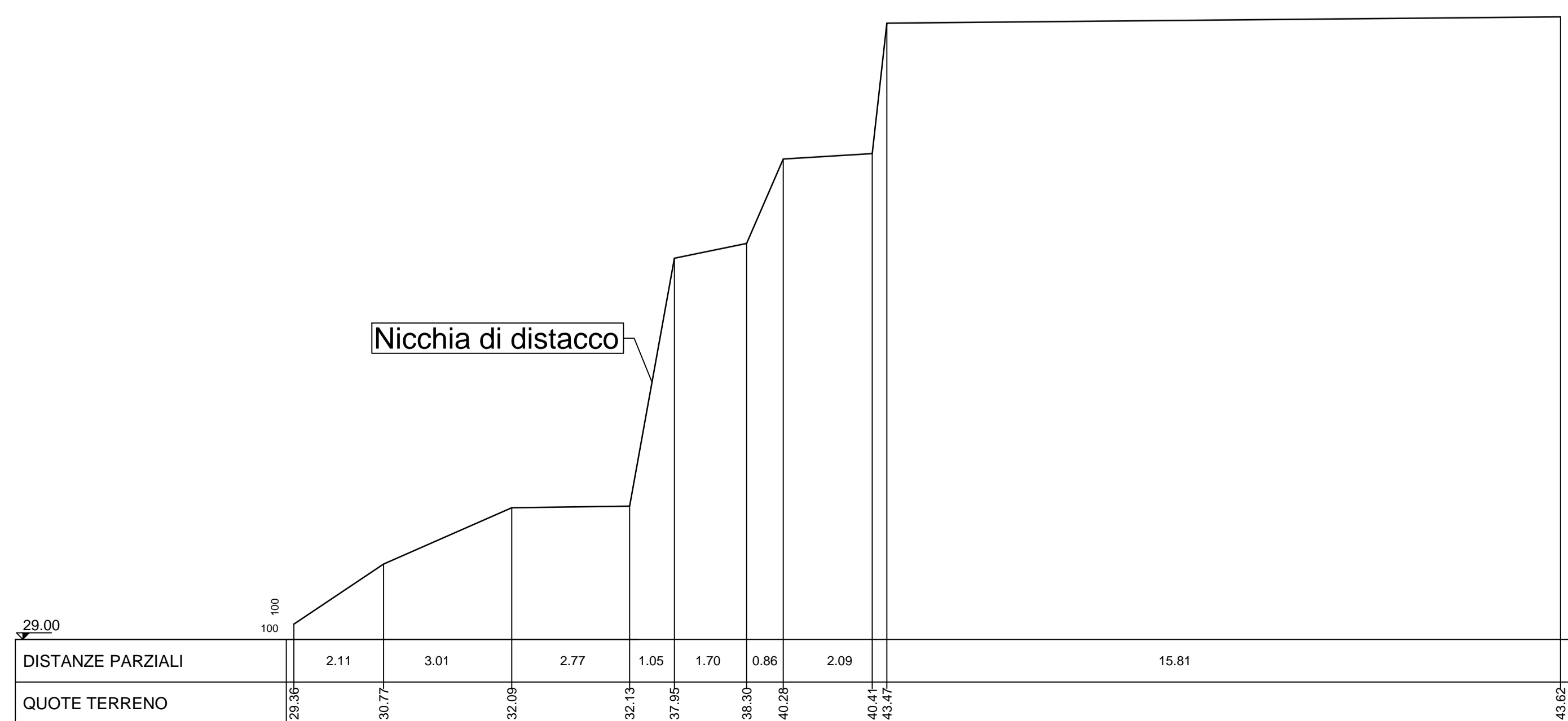
SEZIONE B - B
